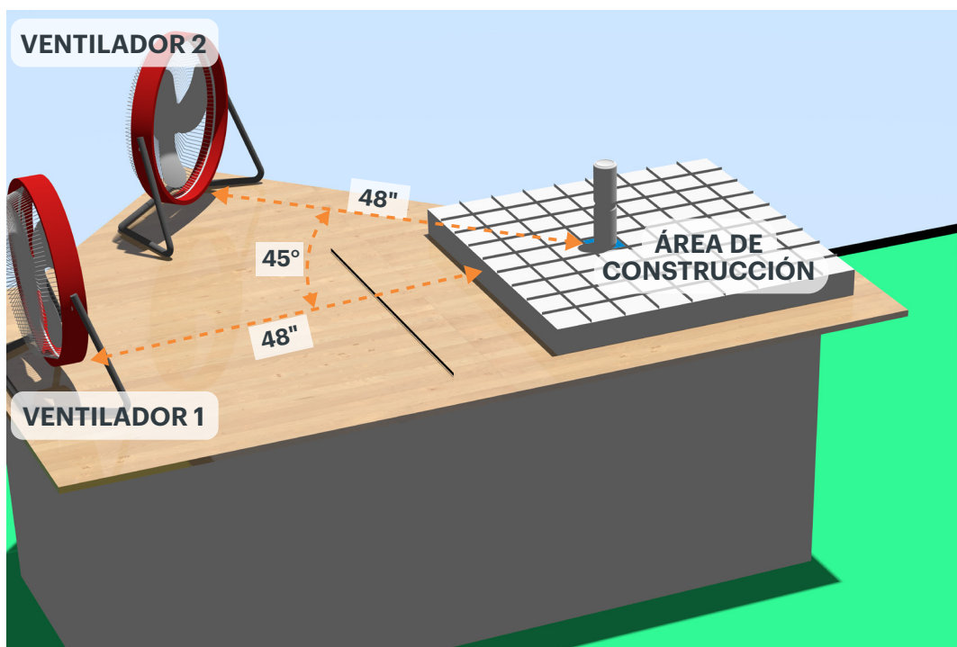
Figura 1: Diagrama de la plataforma (Posición del área de construcción para los grados 4 a 8)
